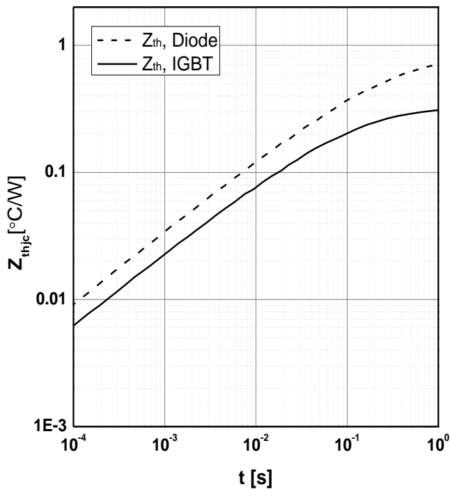
Fig7. Transient Thermal
