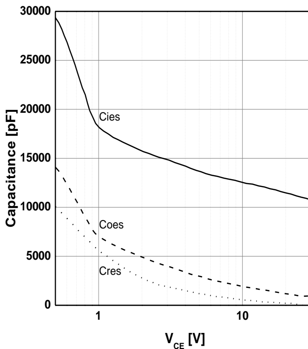
Fig8. Typ. Capacitance
