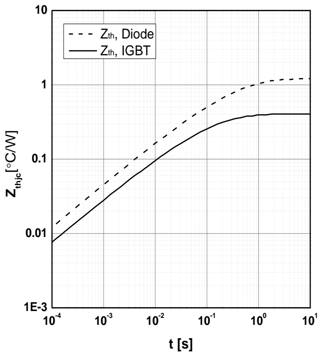
Fig7. Transient Thermal
